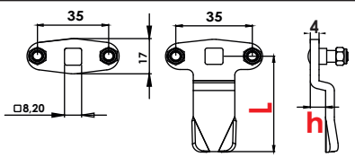
İspanyollet Dilleri Espagnolette Cams
