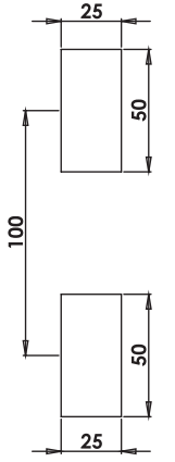
Geçiş Ölçüsü Cut Out
